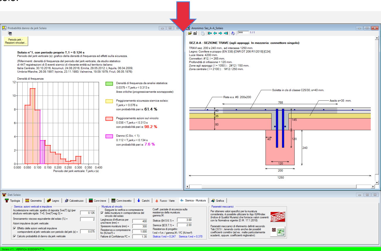
Aedes.SLC: Analisi degli effetti delle azioni sismiche impulsive sul nodo solaio - parete muraria
