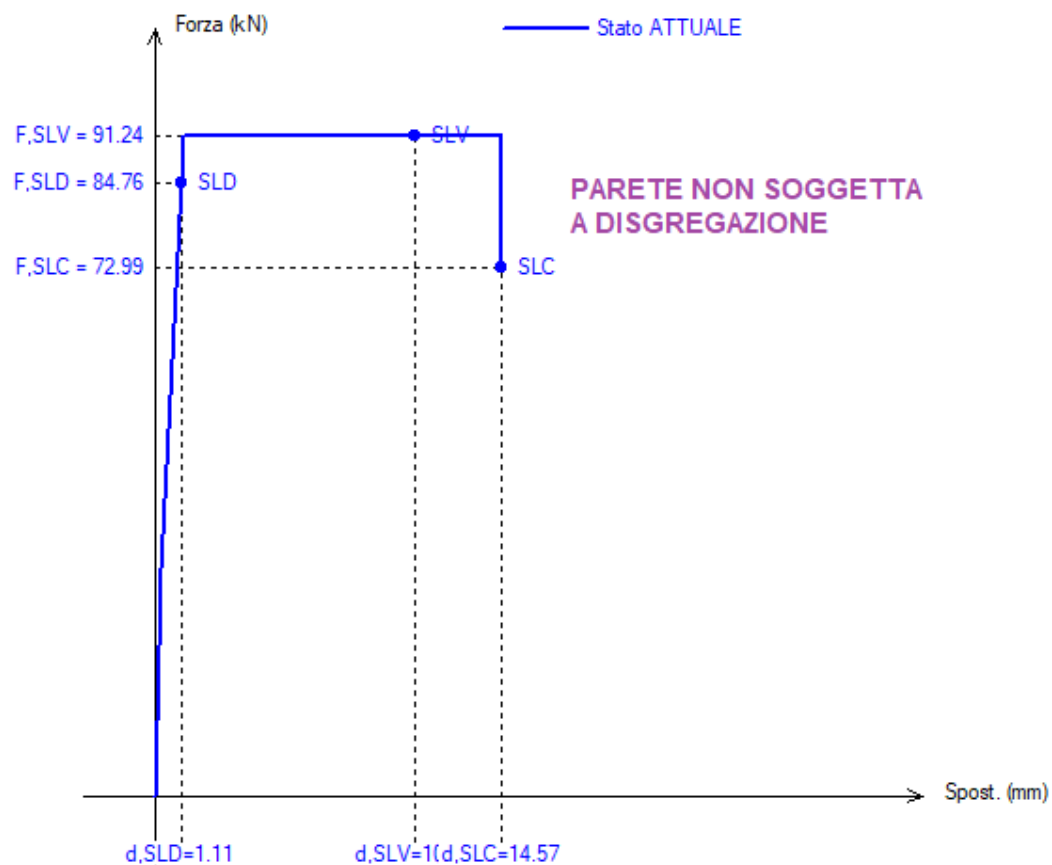
Curva di capacità Parete n° 3 (di 6) - Analisi nel verso +X
