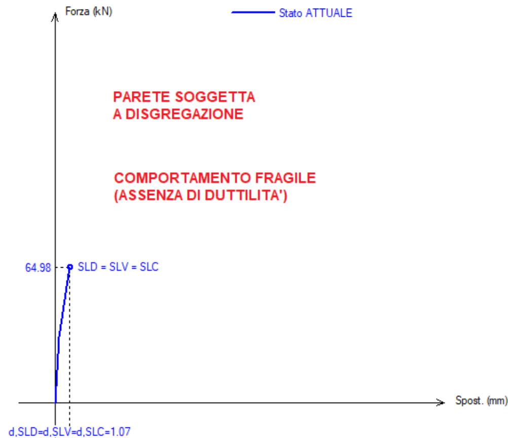
Curva di capacità Parete n° 6 (di 6) - Analisi nel verso +X
