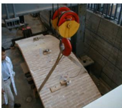
Modalità di imposizione della deformata iniziale sulla volta integra ad un quarto della luce: innalzamento della volta per consentire le vibrazioni libere [1] [2]
